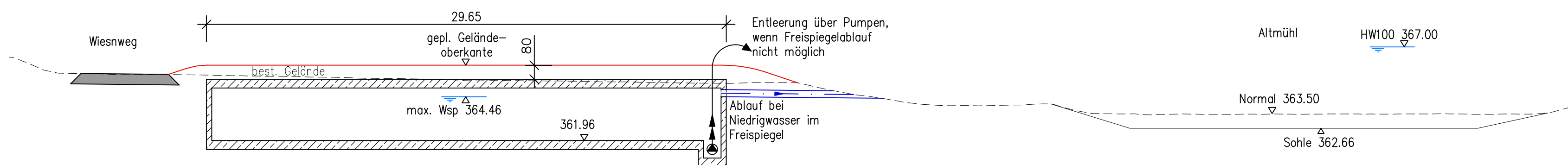
Schnitt B-B M 1:200
